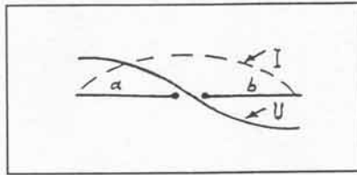
Abb. 1: Strom- und Spannungsverteilung in einer Dipol-Antenne.
